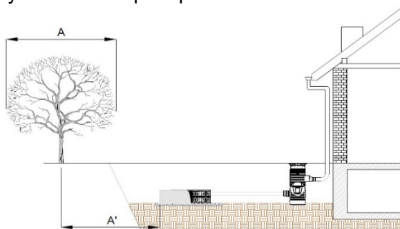
Obrázek 3: Situace instalace: Vzdálenost od stromům
