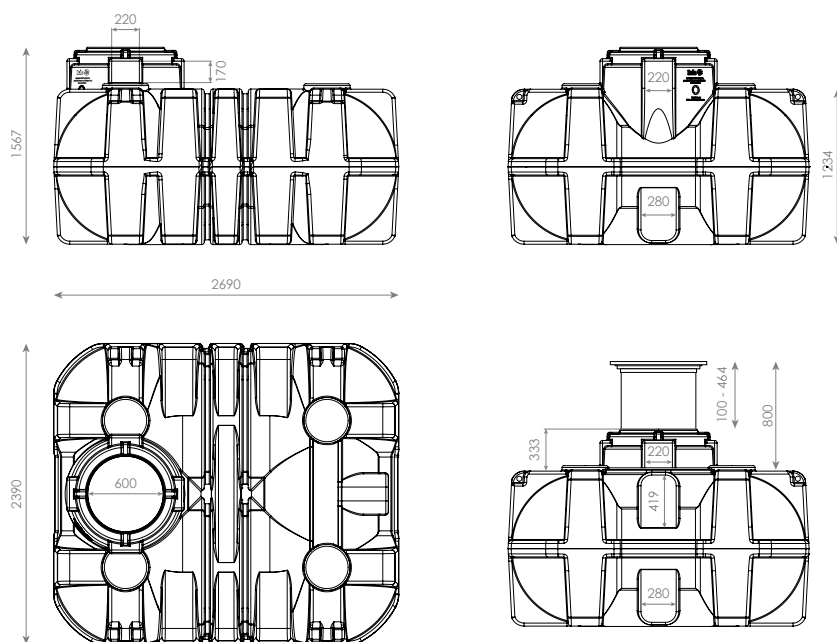
Obrázek 1 - Rozměrový výkres podzemní nádrže Iris 6000
