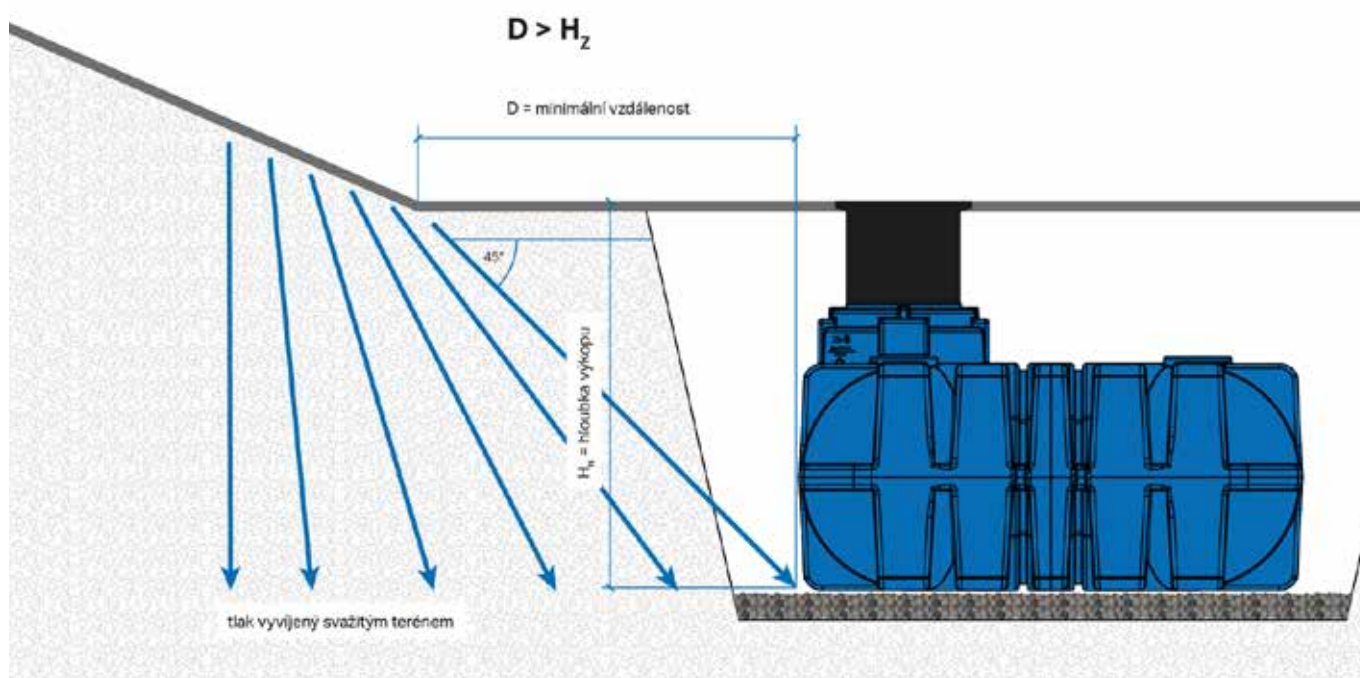
Obrázek 8 - Umístění nádrže ve svahu
