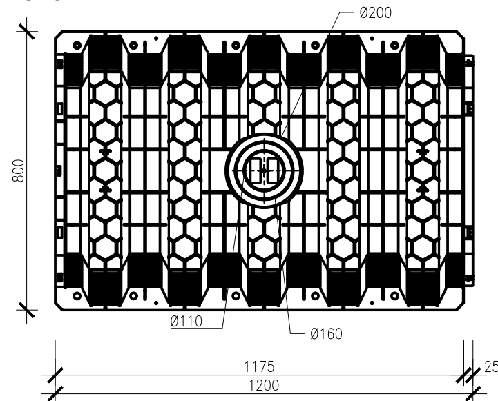
PUDORYS
