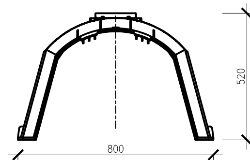
ŘEZ - PŘÍČNÝ
