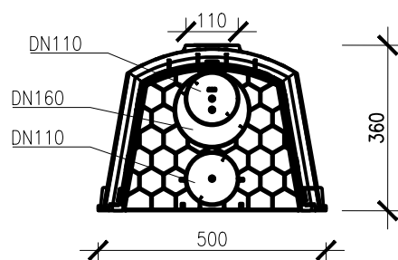
ŘEZ - PŘÍČNÝ (ČELO)
