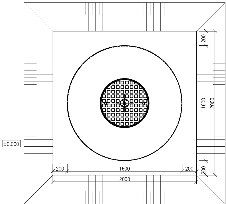
PŮDORYS
